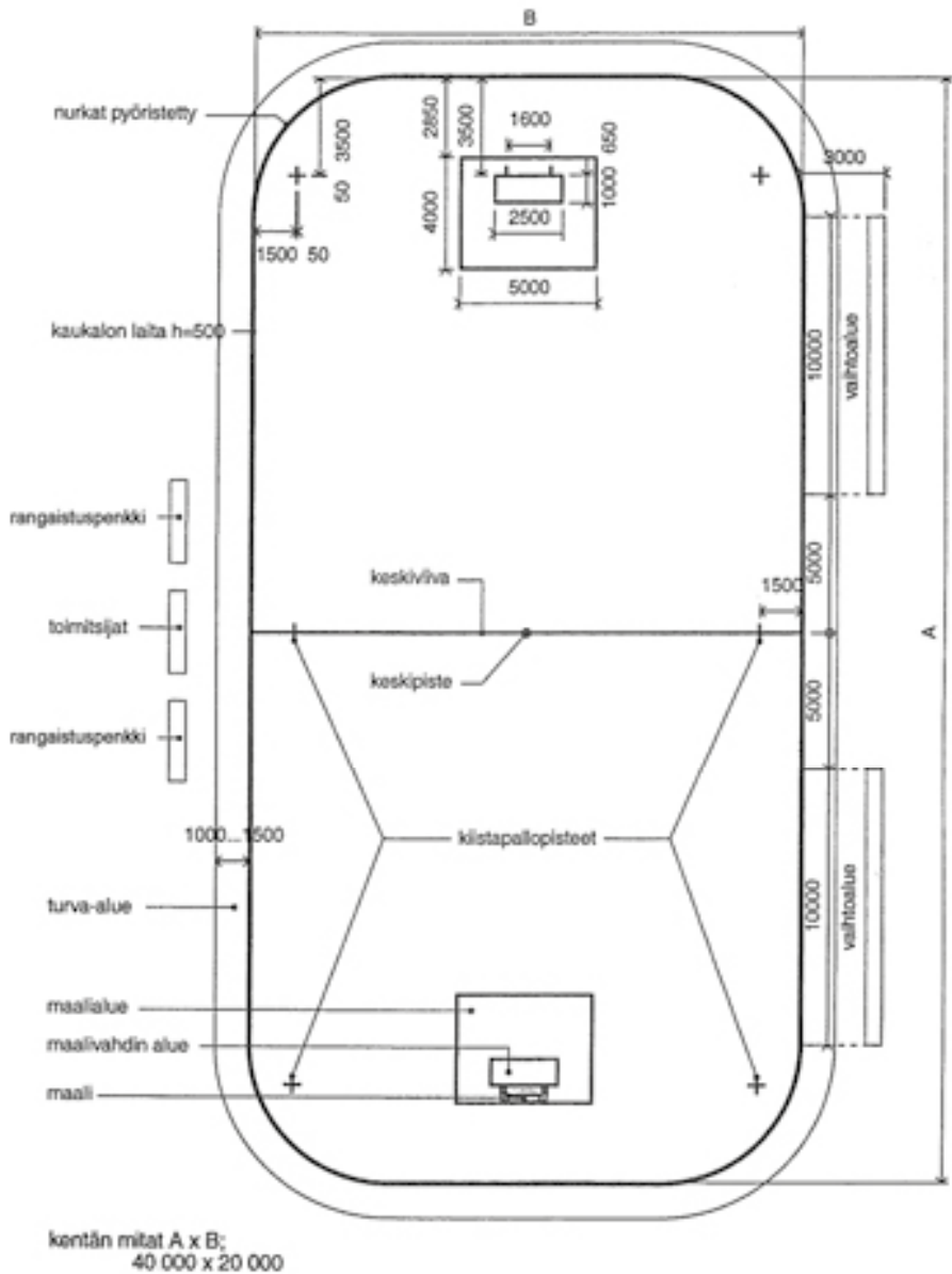
Liite 1. Salibandykentän mitat ja viivamaalaukset
