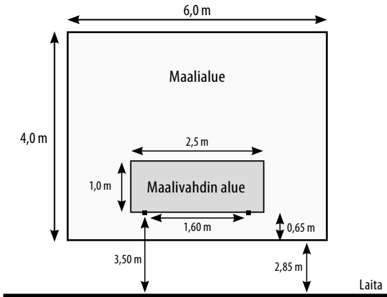
Liite 2. Maalialueen mitat
